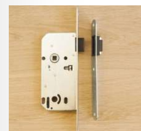
Serrure magnétique avec gâche
